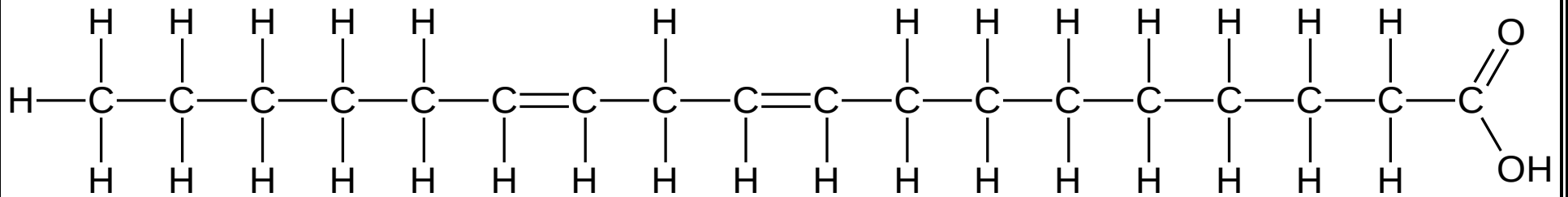
Linolsäure
