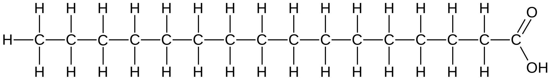
Palmitinsäure
