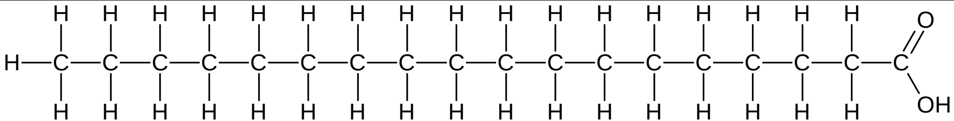
Stearinsäure
