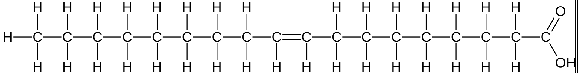
Ölsäure
