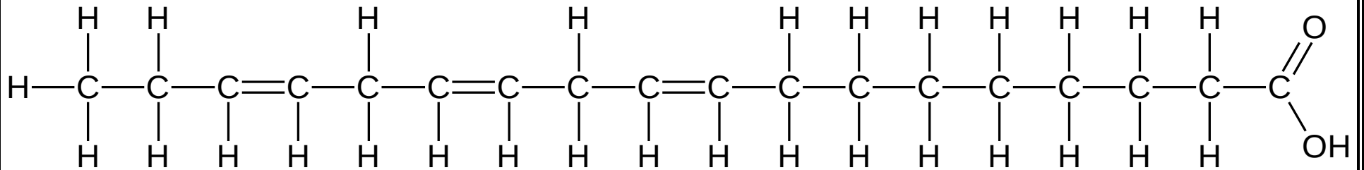
Linolensäure
