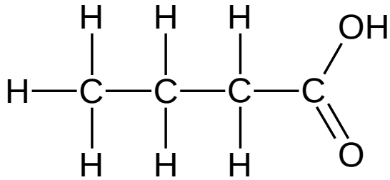
Buttersäure
