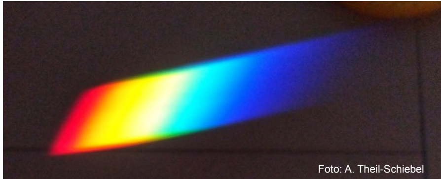
Abb. 1: Farbspektrum
