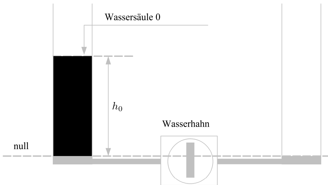
Im Endzustand hat sich das Wasser der Wassersäule 0 in zwei Wassersäulen mit gleicher Masse m_1 = m_0/2 und gleicher Schwerpunkthöhe h_s = h_1/2 = h_0/4 aufgeteilt (siehe Abbildung 4).
